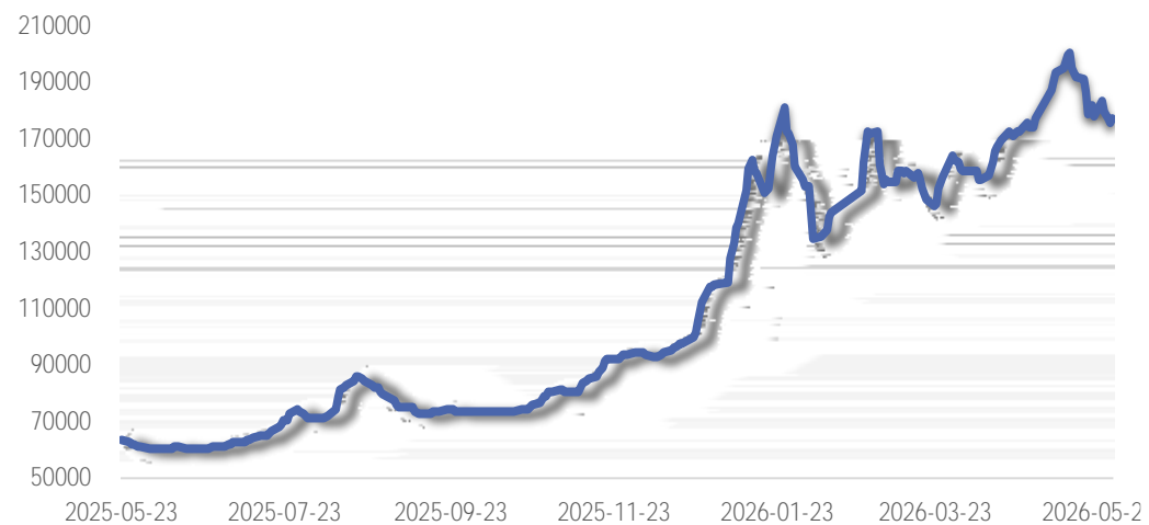
(Li2CO3 99.5%)
