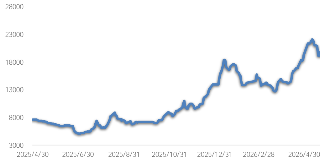
(Li 2 O:7%-8%)
